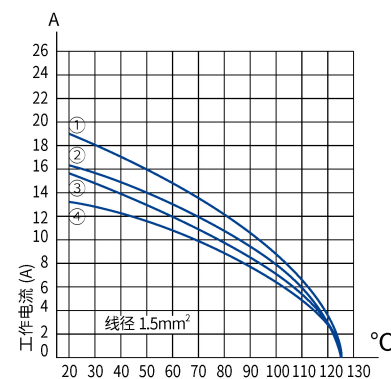
Ambient temperature (°C) 环境温度 (°C) ① HDC-HE6-MS/FS ② HDC-HE10-MS/FS ③ HDC-HE16-MS/FS ④ HDC-HE24-MS/FS
