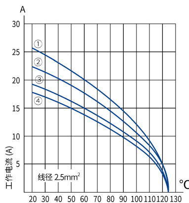
Ambient temperature (°C) 环境温度 (°C) ① HDC-HE6-M/F(MC/FC) ② HDC-HE10-M/F(MC/FC) ③ HDC-HE16-M/F(MC/FC) ④ HDC-HE24-M/F(MC/FC)
